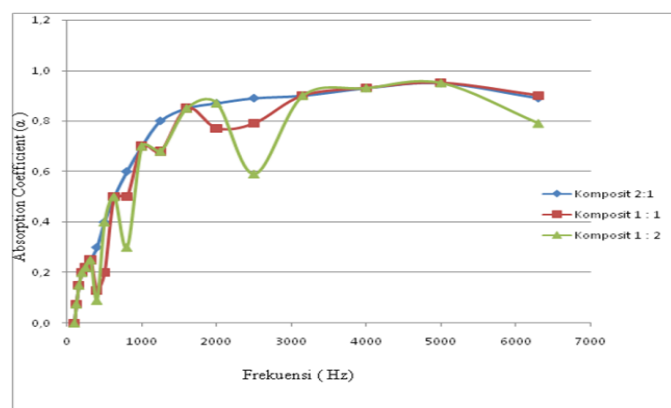
Drawing 3. Frekuensi ( Hz ) dengan Absorption Coefficient ( \alpha )
