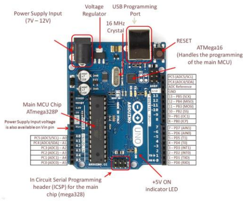
Fig 3: Arduino Uno
