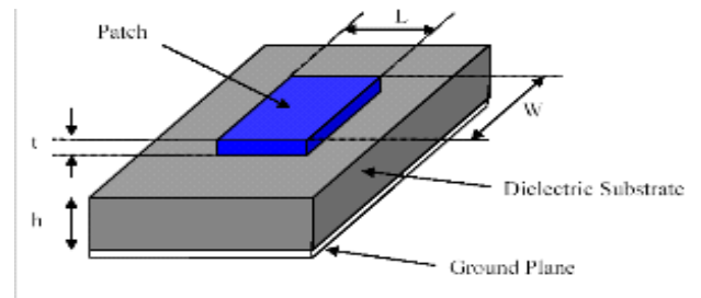
Fig.1. Microstrip Antenna
