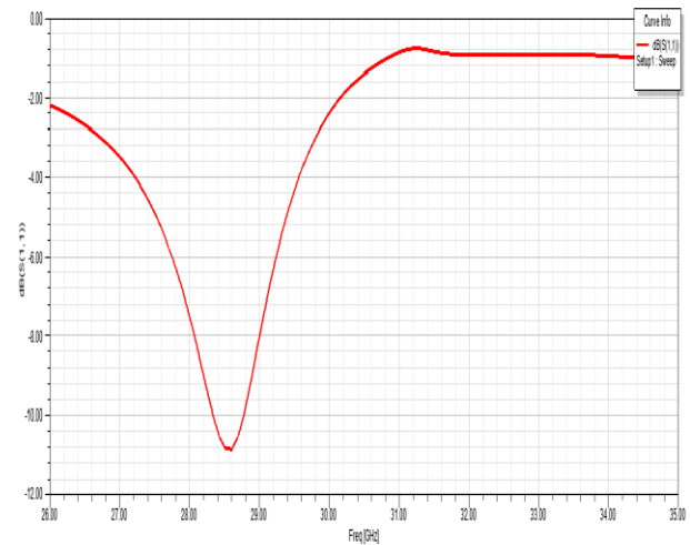
Fig 5. S Parameter values of linear array antenna
