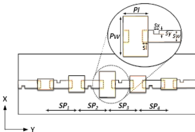
Fig1. 1×5 array antenna
