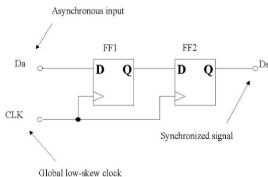
Fig. 1 Synchronizer
