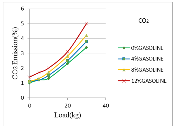
CO2 Emission Vs Load
